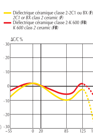
Fig. 89 Variation relative de la capacité en fonction de la température. Relative capacitance change vs temperature.
