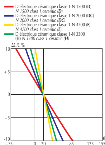
Fig. 88 Variation relative de la capacité en fonction de la température. Relative capacitance change vs temperature.
