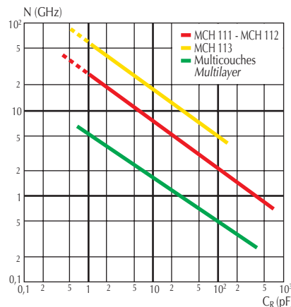
Fig. 86 Fréquence de résonance série. Resonant series frequency.
