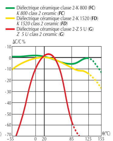
Fig. 90 Variation relative de la capacité en fonction de la température. Relative capacitance change vs temperature.
