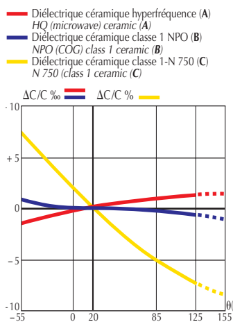
Fig. 87 Variation relative de la capacité en fonction de la température. Relative capacitance change vs temperature.
