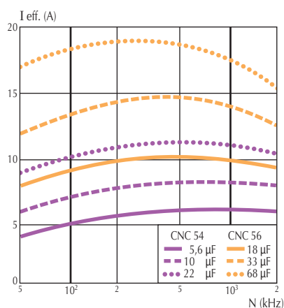
Fig. 72 bis. Intensité efficace en fonction de la fréquence U_{RC} = 63 V_{CC} ( \Delta\theta 20°C). Permissible RMS current vs frequency.
