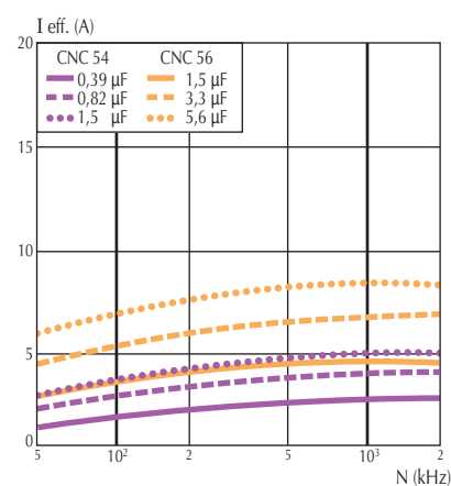
Fig. 75 bis. Intensité efficace en fonction de la fréquence U_{RC} = 500 V_{CC} ( \Delta\theta 20^{\circ}C ). Permissible RMS current vs frequency.
