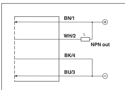
Uscita NPN DECOU ® DECOU ® output NPN
