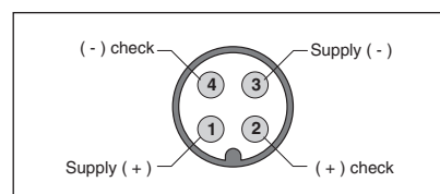
M12 Emittitore con check Emitter with check
