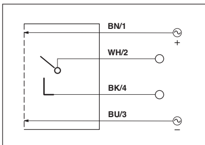
Uscita NPN DECOU ® DECOU ® output NPN
