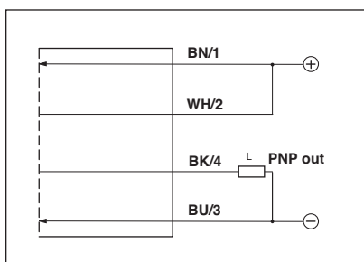
Uscita PNP DECOU ® DECOU ® output PNP
