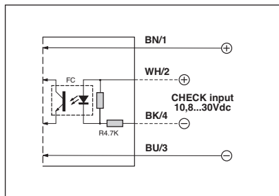
Emettitore con check Emitter with check
